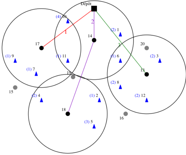
FIGURE 6: Solution du CTP-CCVRP avec deux camions disponibles. Le résultat du CTP-VRP étant le même pour deux, trois et quatre camions, on se référera à figure 4.
