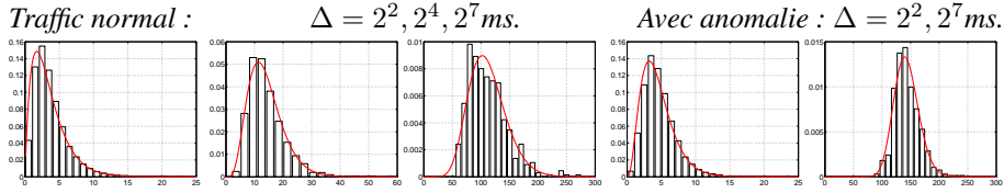
Figure 3. Marginales du trafic et Lois Gamma. Distributions marginales du trafic agrégés à différents niveaux différents et ajustés par des lois \Gamma_{\alpha,\beta} . À gauche : trafic normal ( \Delta = 2^2, 2^4, 2^7 ms). À droite : trafic pendant l'attaque III ( \Delta = 2^2, 2^7 ms).
