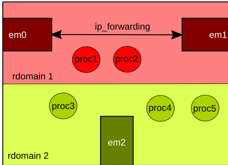
Figure 3 - Exemple de domaines de routage
