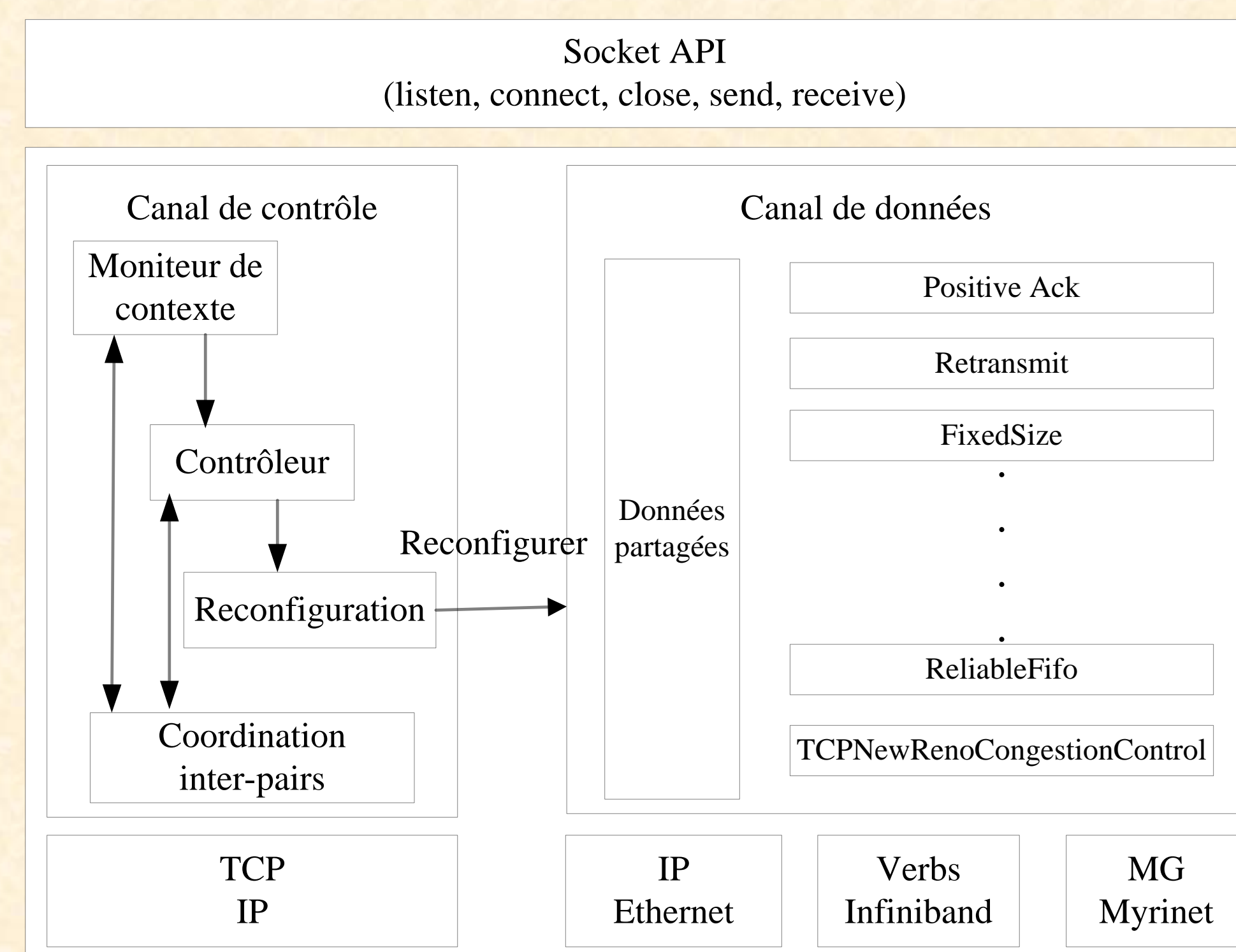
Architecture du protocole auto-adaptatif
