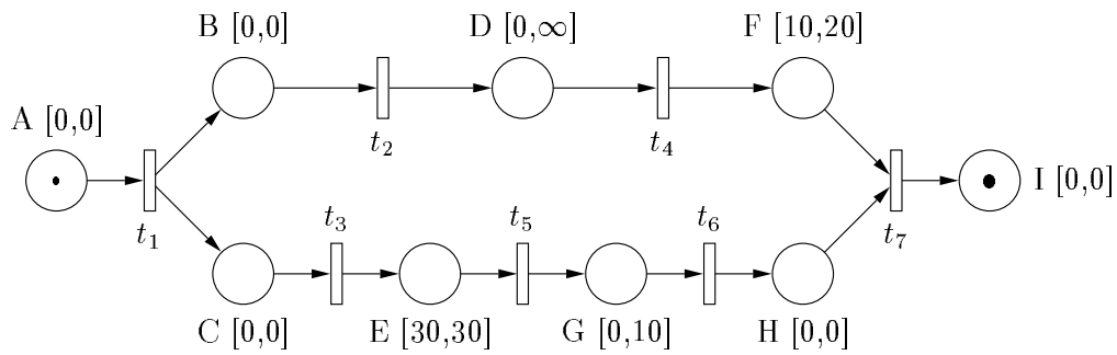
FIG. 4: Réseau de Petri P-temporel
