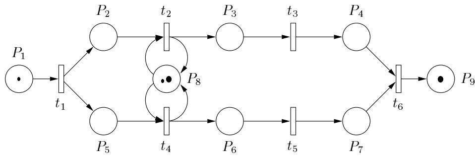
FIG. 1: Réseau de Petri avec conflit
